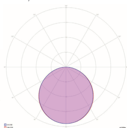
vyzařovací charakteristika
