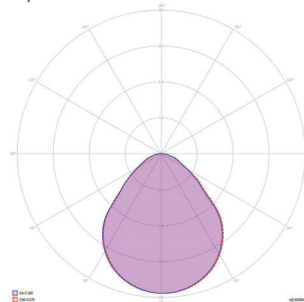
vyzařovací charakteristika
